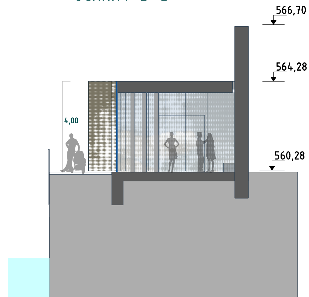
Schnitt C-C
