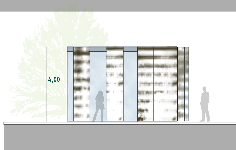
Ansicht West
