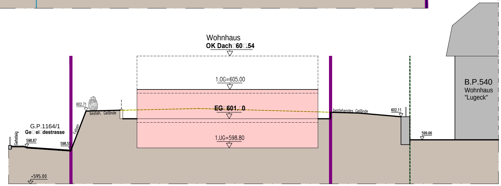
Schnitt/sei 3:3
