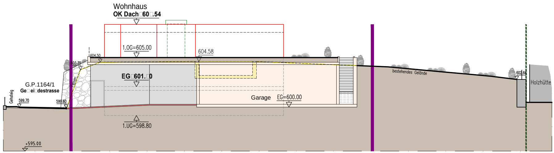
Schnitt/sei 1:1
