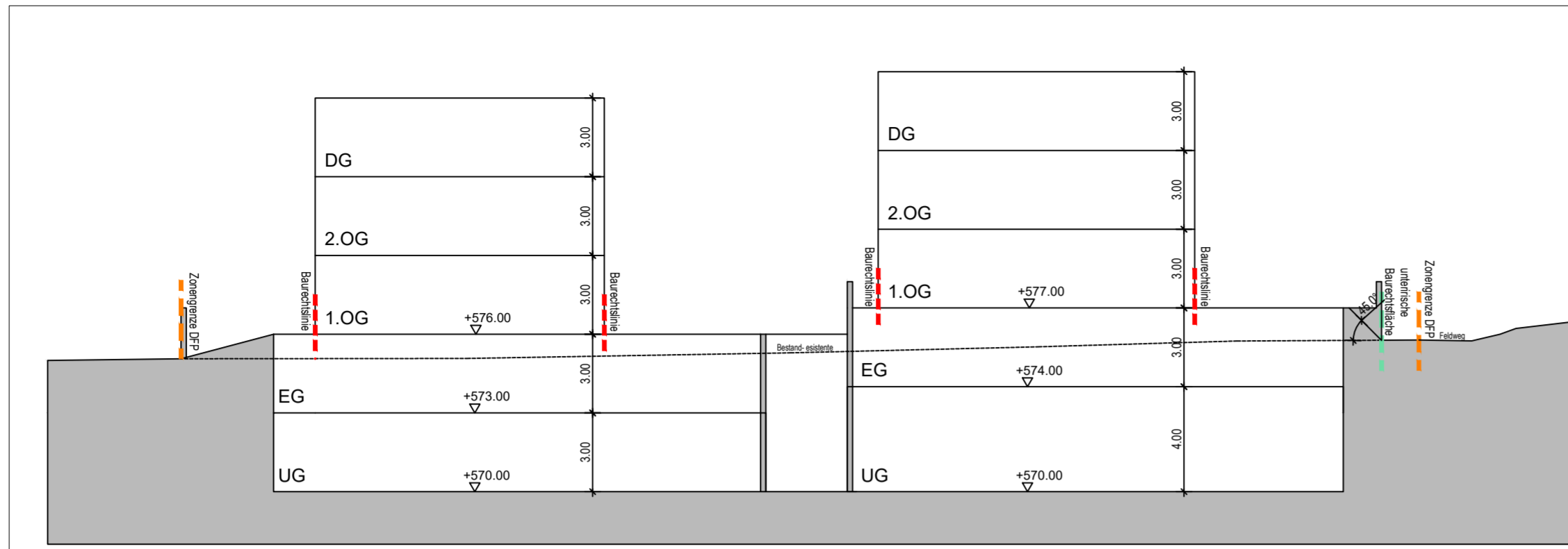
schnitt E- sezione E 1:200
