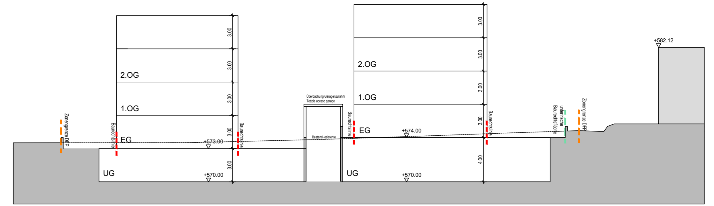
schnitt F- sezione F 1:200
